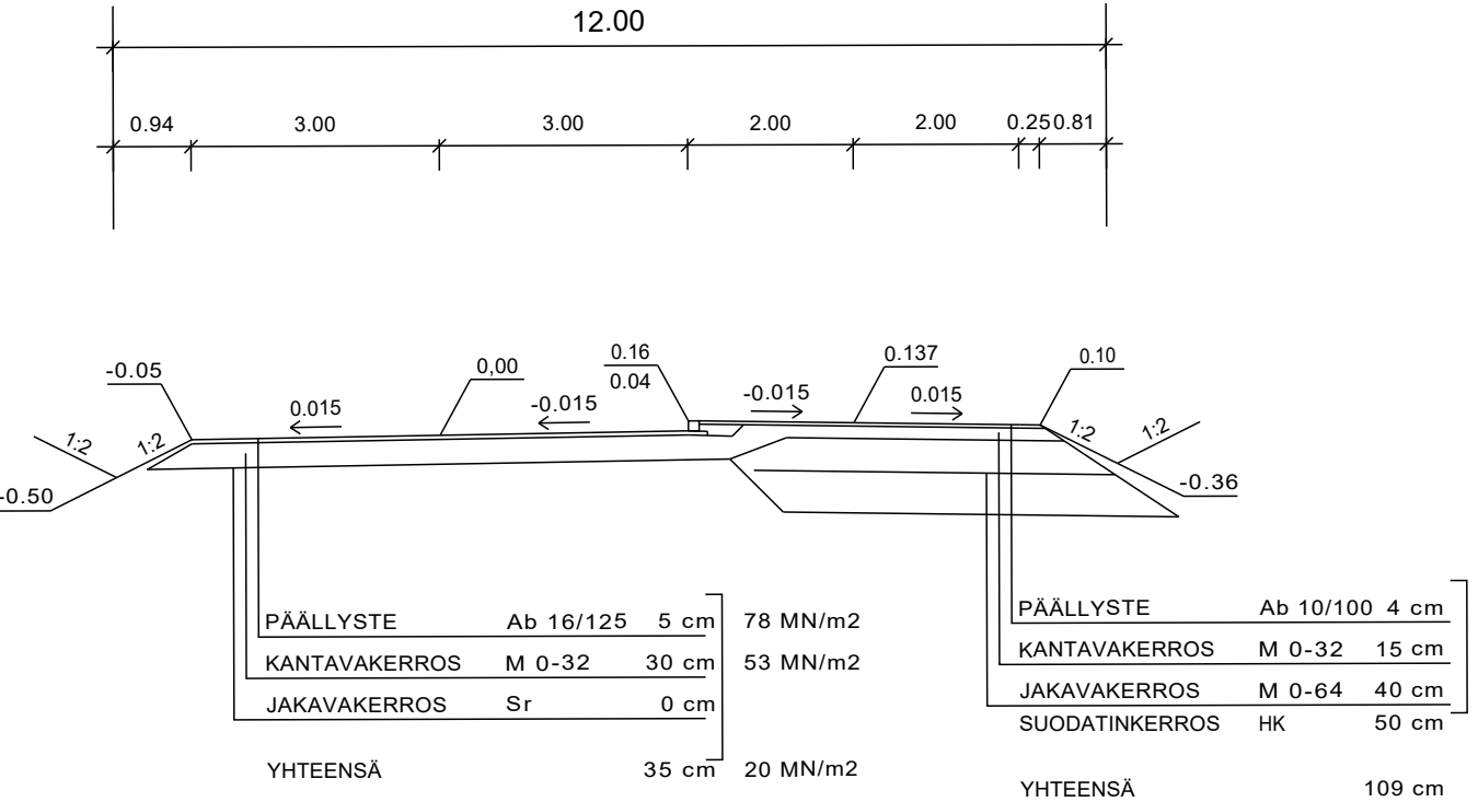
HUOLTOTIE_LEIKKAUS PL 45-90
