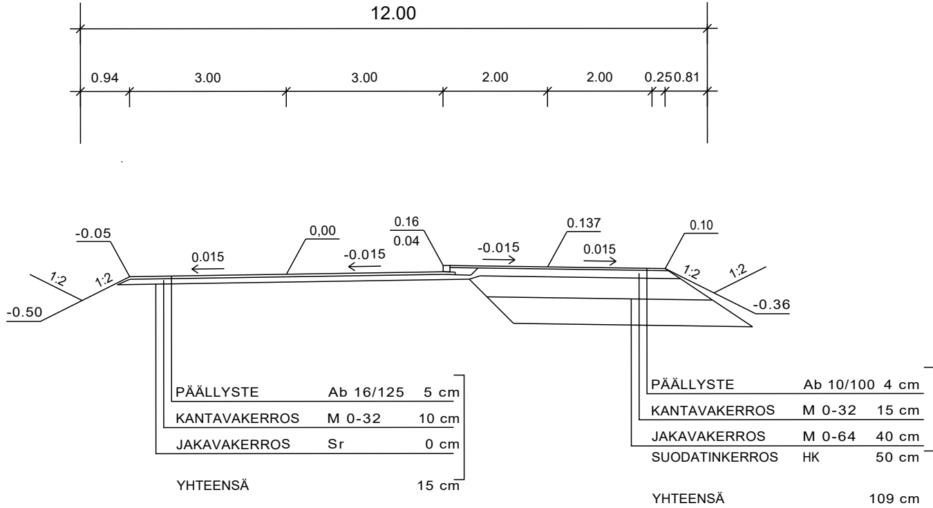
HUOLTOTIE_LEIKKAUS PL 45-90
